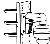
DS-1275ZJ-SUS Кронштейн для установки на столб (стойку)
